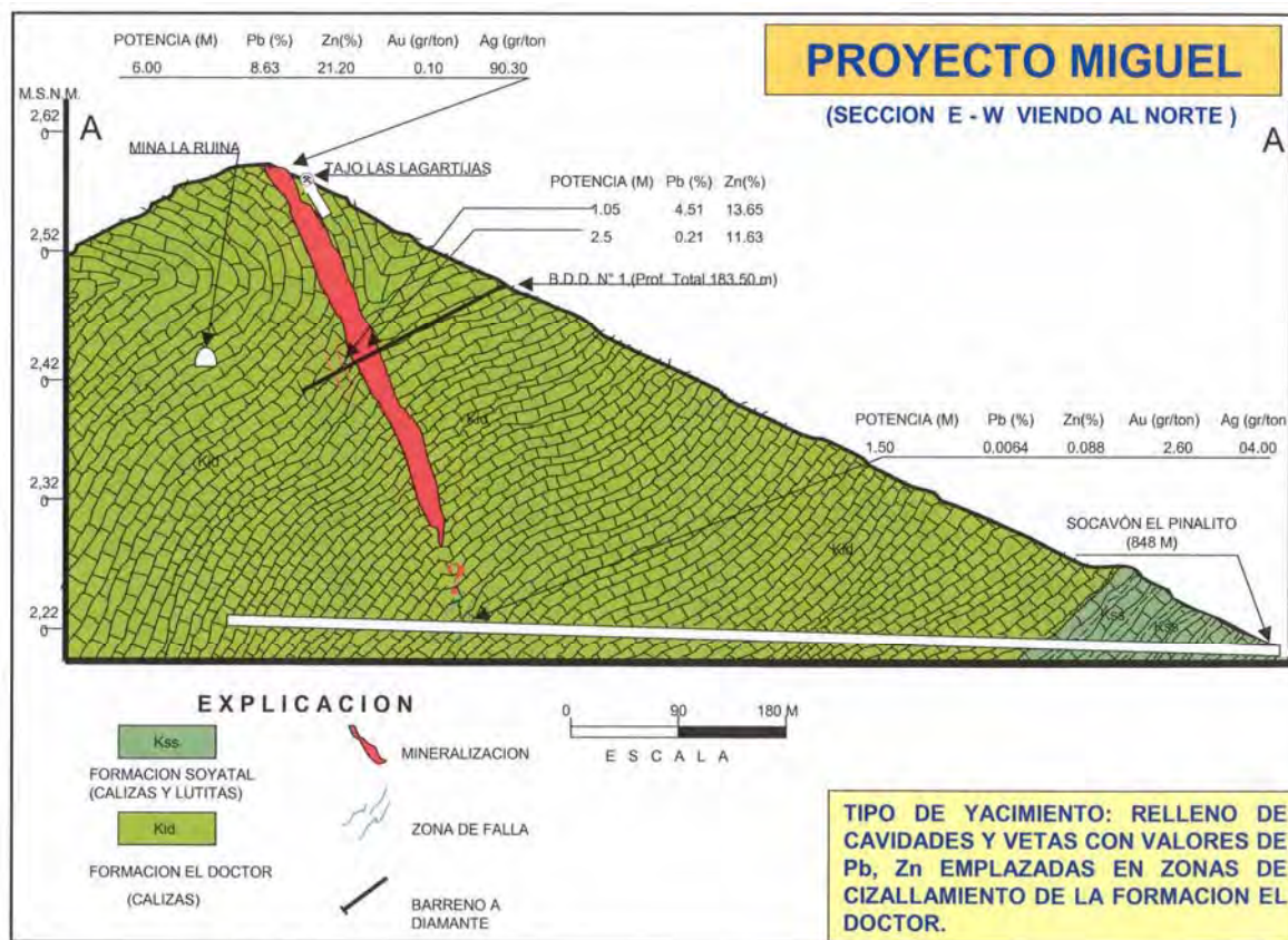
FIG 5.- SECCIÓN GEOLÓGICA Y MUESTREO SOBRE LA ESTRUCTURA MINERALIZADA.
