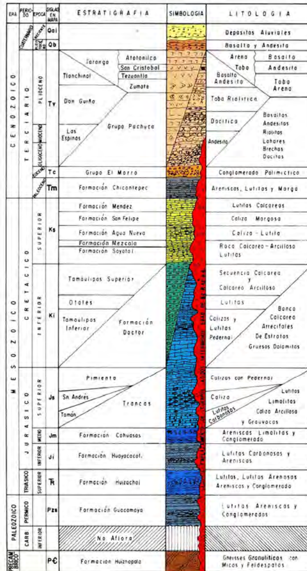
FIG 2.- COLUMNA GEOLOGICA
