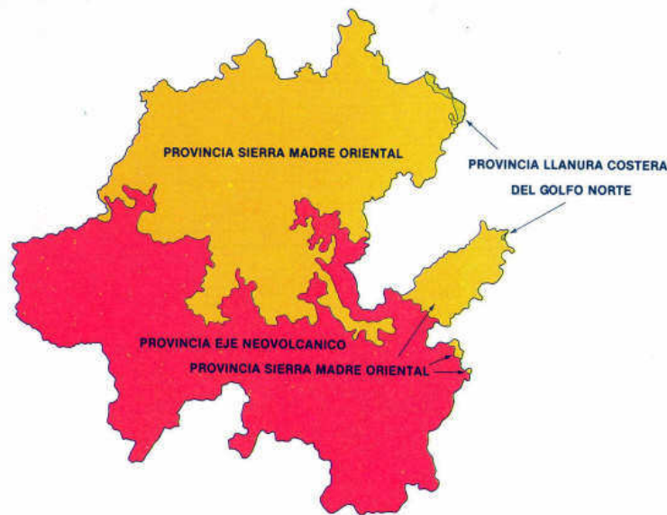
Fig. 1.- Provincias fisiográficas del estado de Hidalgo (cf. INEGI 1999)
